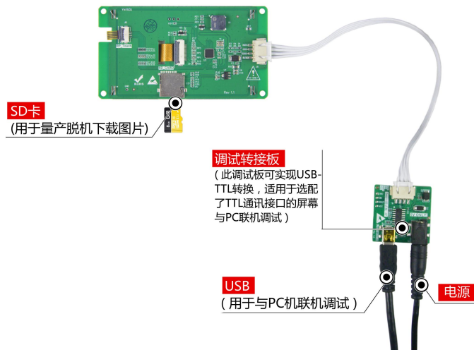
图 1-4 调试工具图
