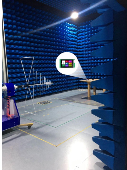
图 4-4 RE 测试图
